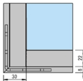
Ansicht innen
