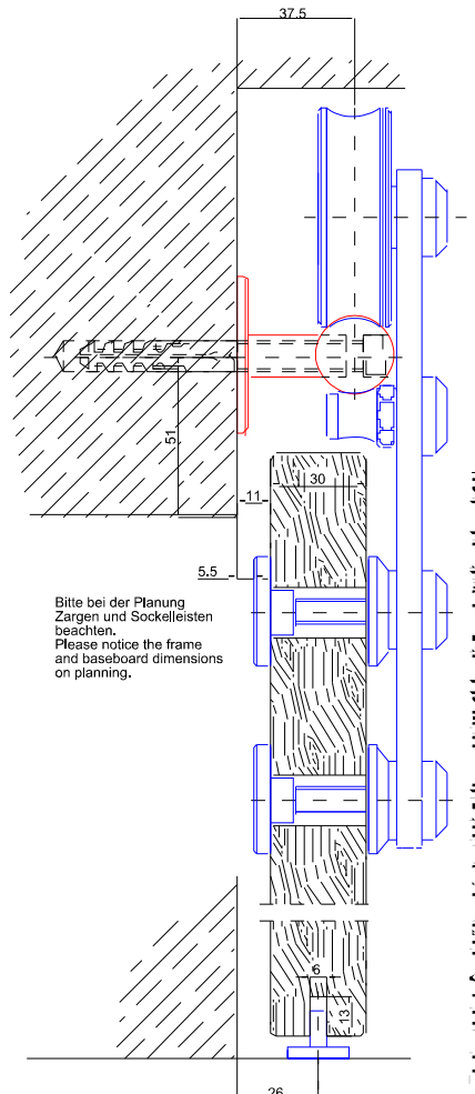
Beispiel mit 30mm Holz Türblatt example with 30mm wooden door
