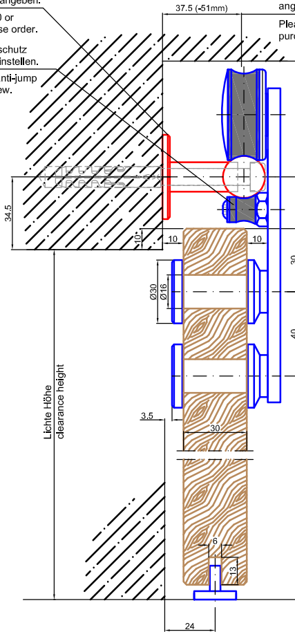
Beispiel mit 30mm Holztürblatt example with 30mm wooden door
