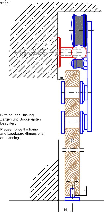
Beispiel mit 20mm Holztürblatt example with 20mm wooden door
