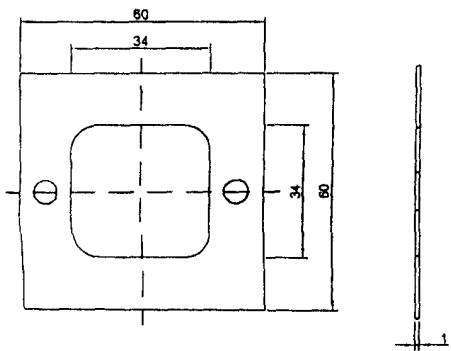
Zwischenlage
