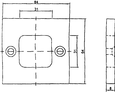
Vorderseite
